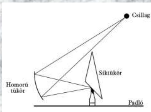
XLIV. ábra: A tükrök elrendezése a káldeai templomban
